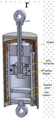
MR Sönümleyici
